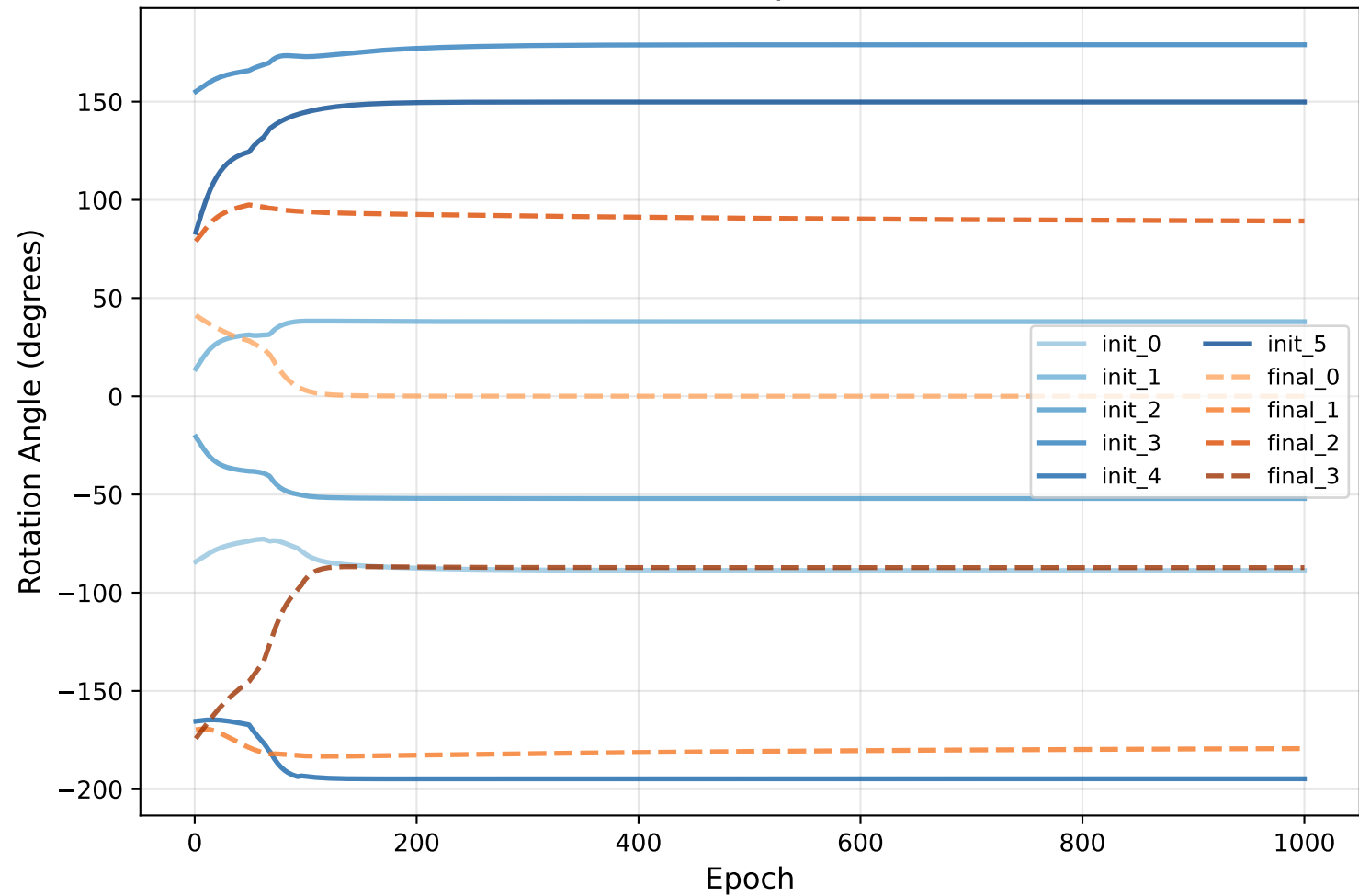
Parameter Evolution (10 params: 6 init, 4 final)
